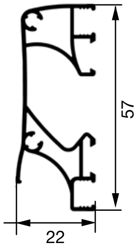
Querprofil
