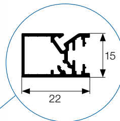
Unteres Rahmenprofil
